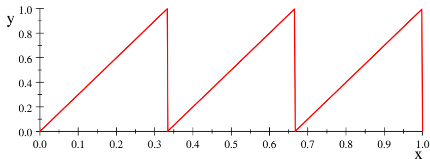
Wykres p_{\lfloor \pi \rfloor}(x,)
